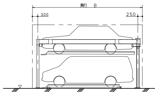
側面図
