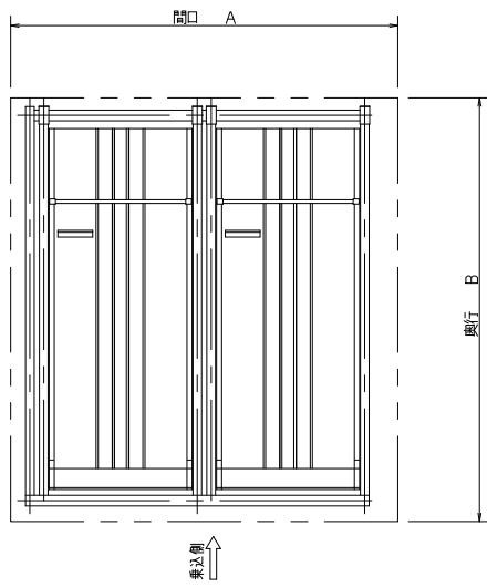
平面図
