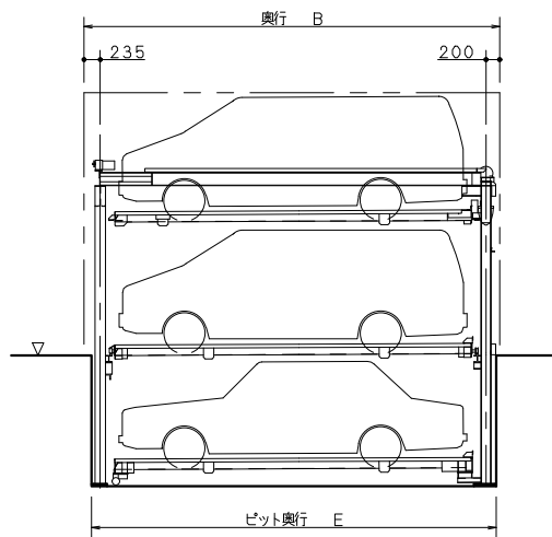
側面図
