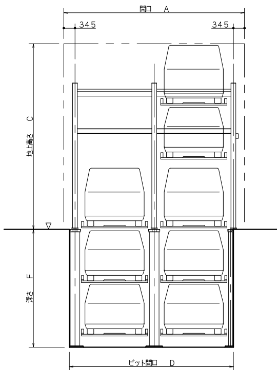
正面図
