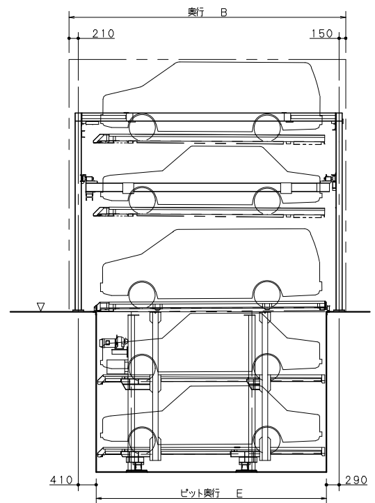
側面図
